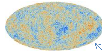
Relevé des fluctuations thermiques de l'univers observées par la mission Planck (mars 2013)
